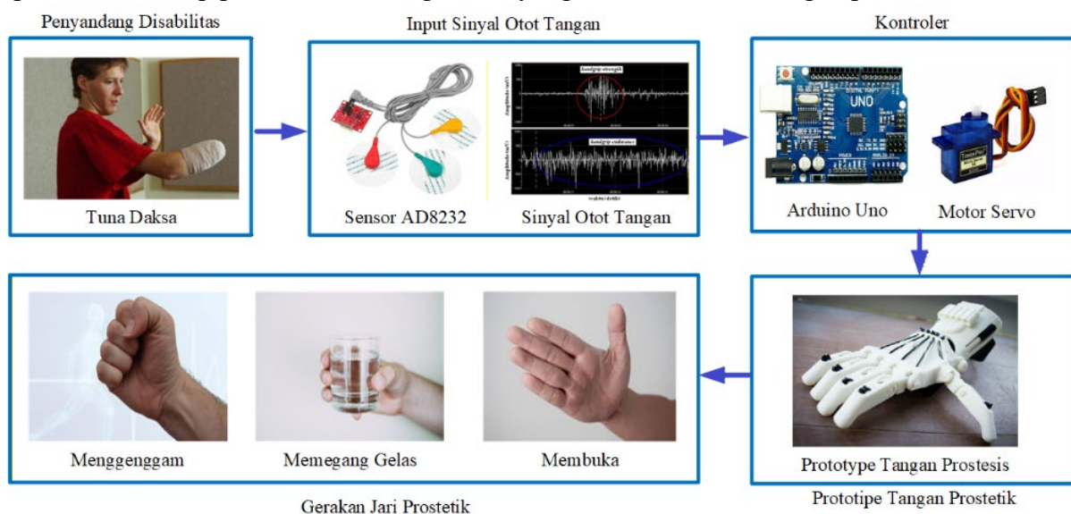
Gambar 1. Desain Penelitian
