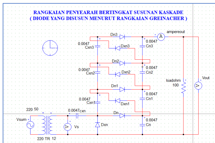
Gambar 2. Rangkaian Simulasi Cascade Greinacher Menggunakan PSIM
