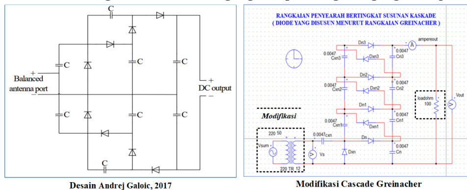
Gambar 1. Modifikasi Desain Cascade Greinacher
