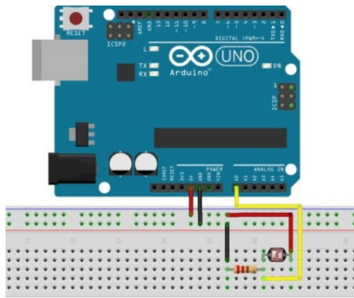
Gambar 1. Rangkaian Sensor LDR
