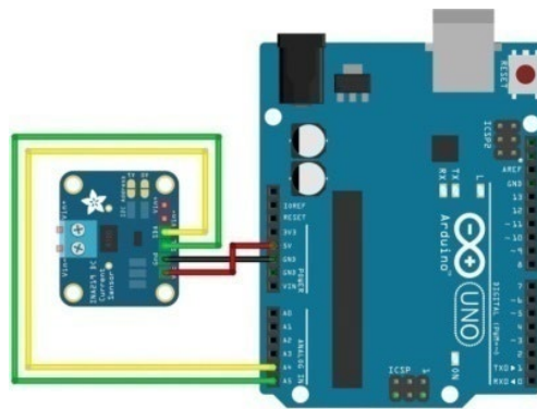
Gambar 2. Rangkain Modul INA219
