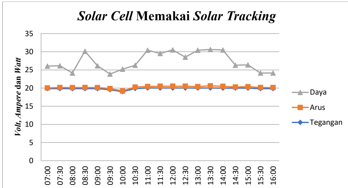
Gambar 5. Grafik Hasil Skenario Pertama Solar Cell Memakai Solar Tracking
