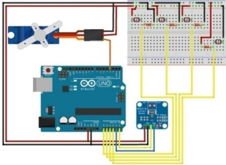
Gambar 4. Konfigurasi Pin Keseluruhan Sistem
