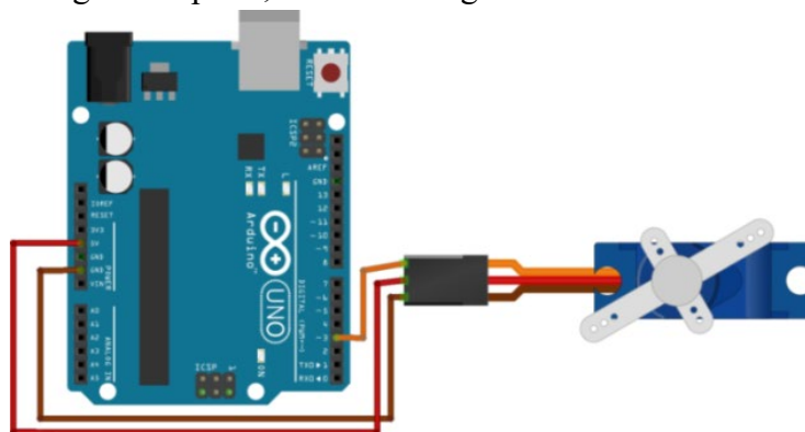
Gambar 3. Rangkaian Motor Servo
