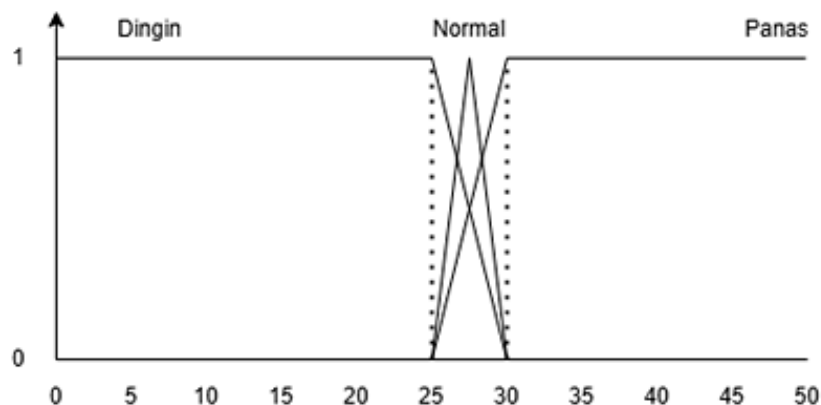
Gambar 6. Fungsi Keanggotaan Variabel Suhu
